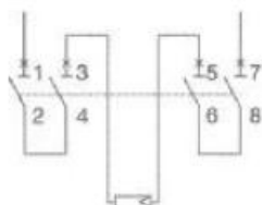
4P 外形
