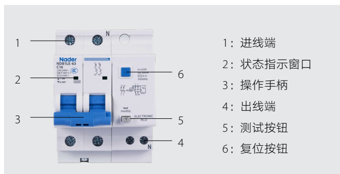
NDB1LE-63 外部结构
