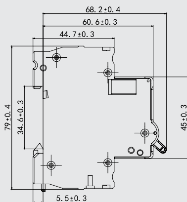
1P侧视图
