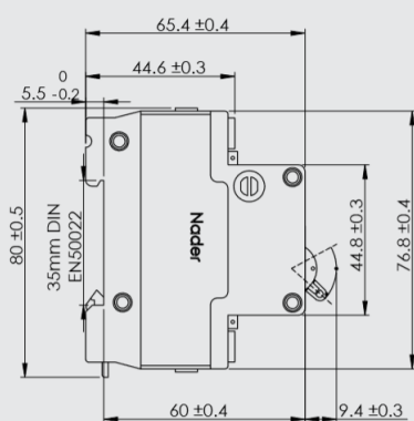
1P侧视图
