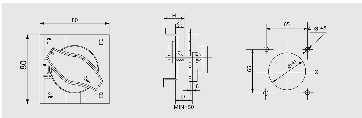
IP65手柄（400壳架以上）开孔示意图
