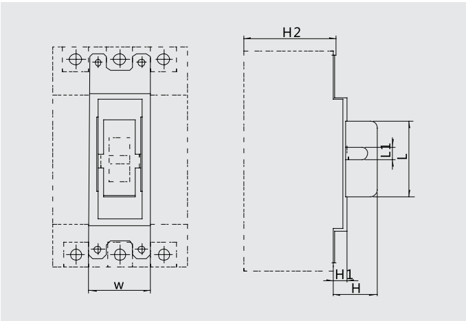
MS1 锁机构安装示意图
