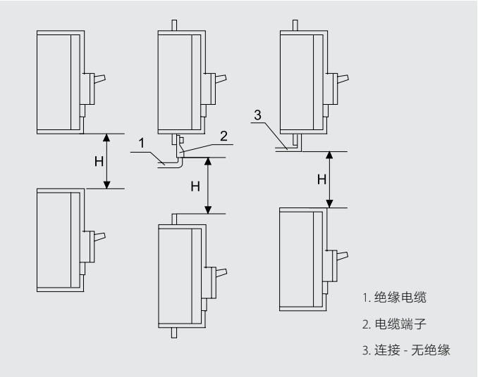
断路器叠装之间最小距离
