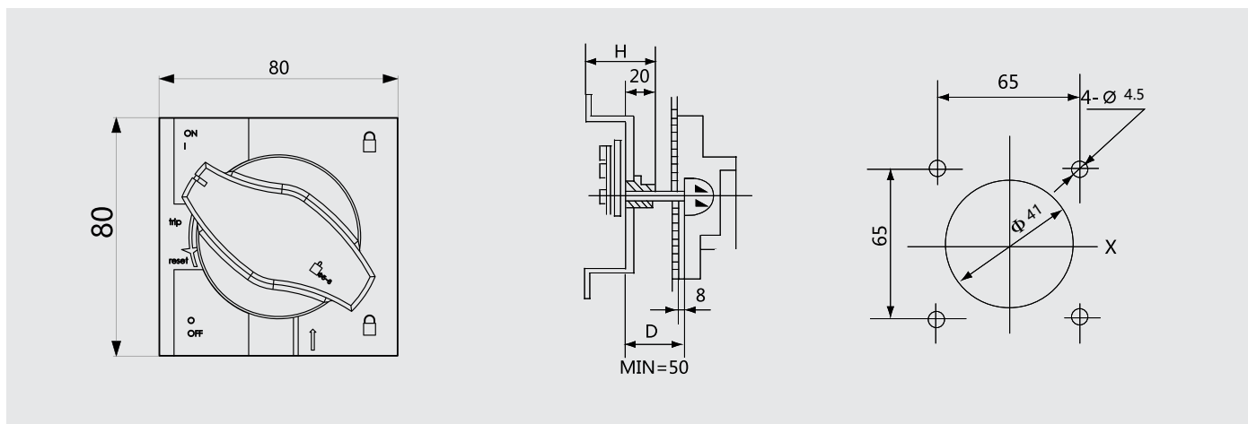
IP65手柄（400壳架以上）开孔示意图
