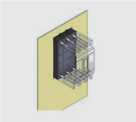
安装示意图：
