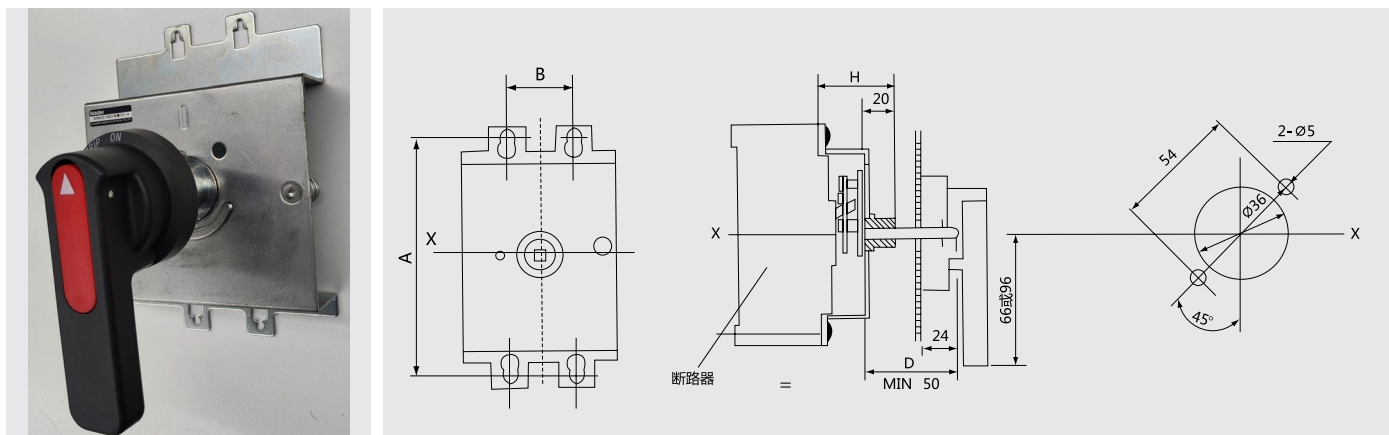
CS1-A型手柄安装开孔示意图
