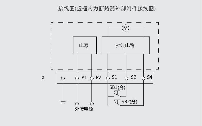
电动操作机构（配用NDM2Z-63~630系列）
