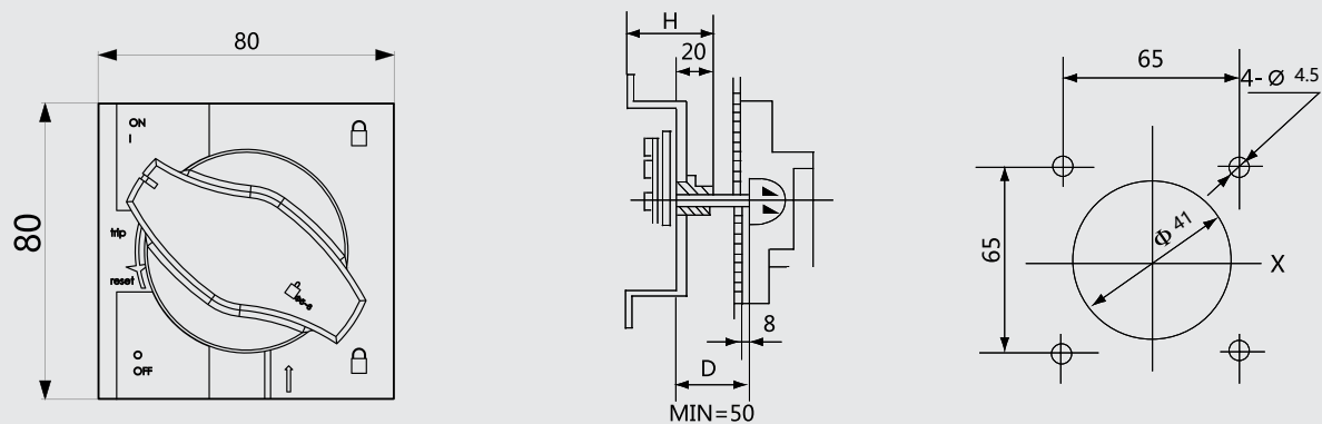
IP65手柄（250壳架以下）开孔示意图
