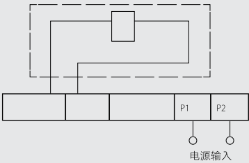
欠压脱扣器接线图
