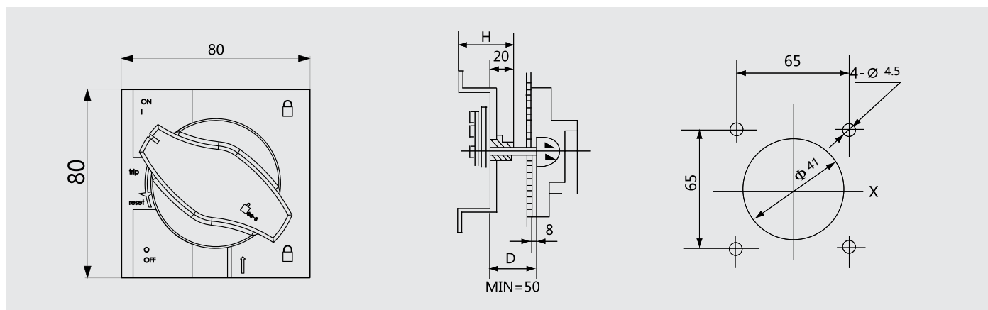
P65手柄（400壳架以上）开孔示意图
