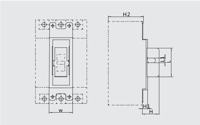
MS1 锁机构安装示意图
