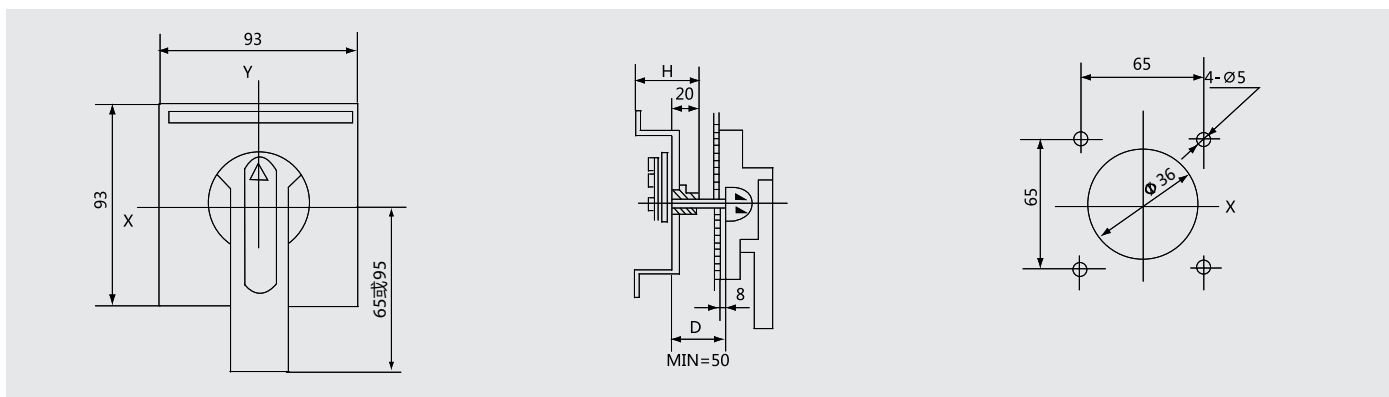
CS1-F型手柄安装开孔示意图
