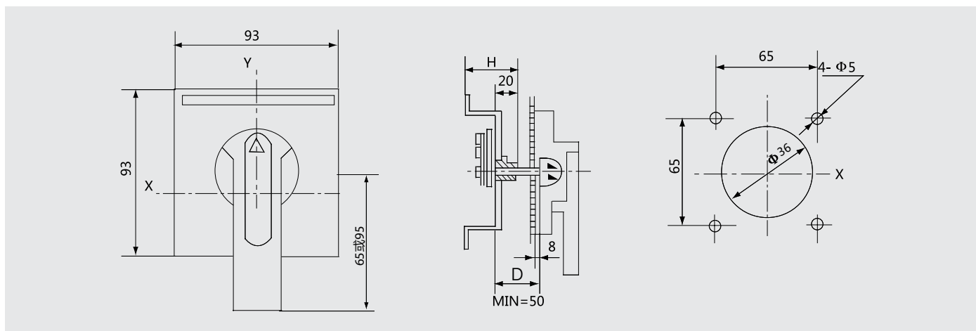
CS2-A型手柄安装开孔示意图
