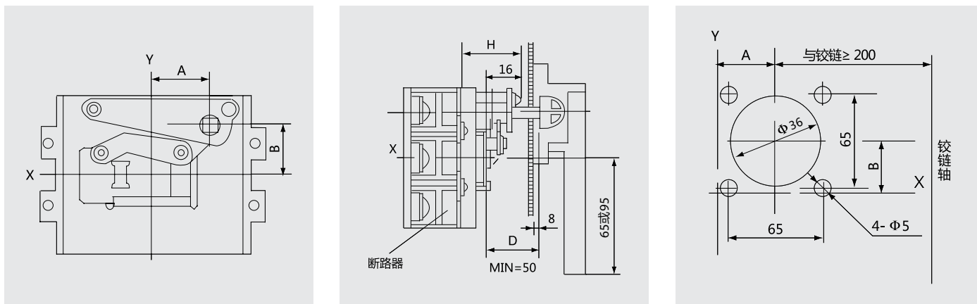
CS2-F型手柄安装开孔示意图
