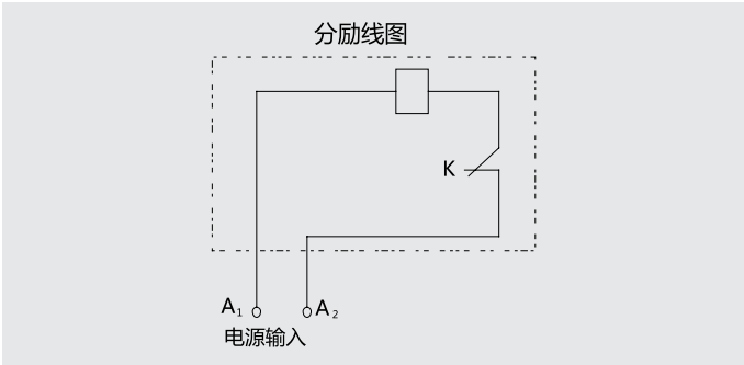
分励脱扣器接线图
