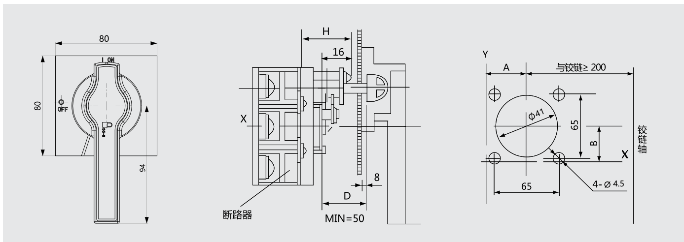
IP65手柄（400壳架以上）开孔示意图
