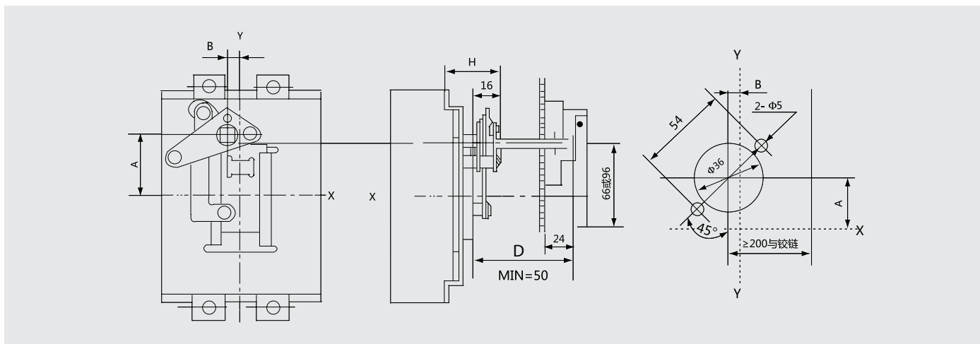
CS2-A型手柄安装开孔示意图
