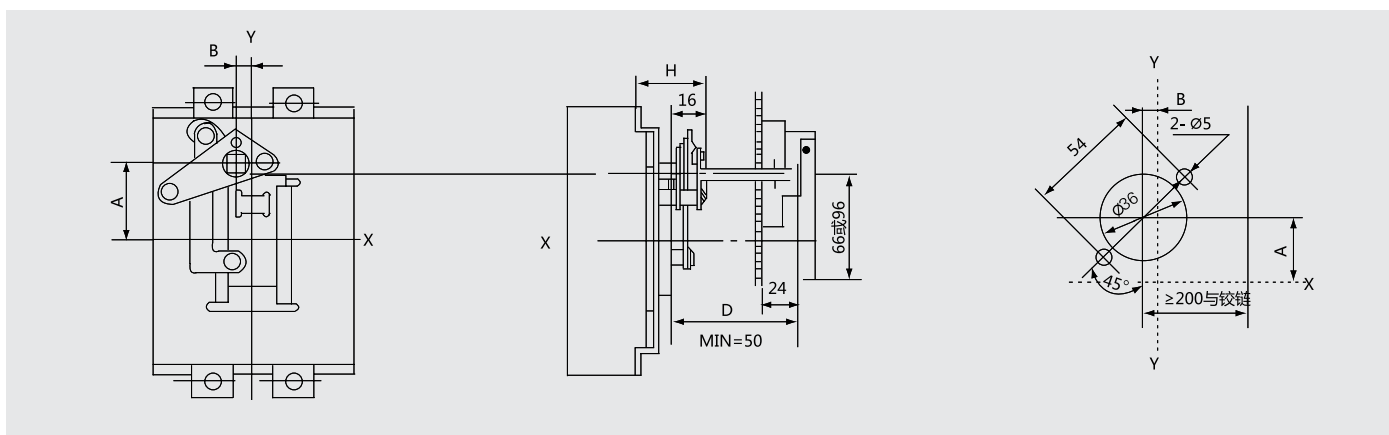
CS2-A型手柄安装开孔示意图
