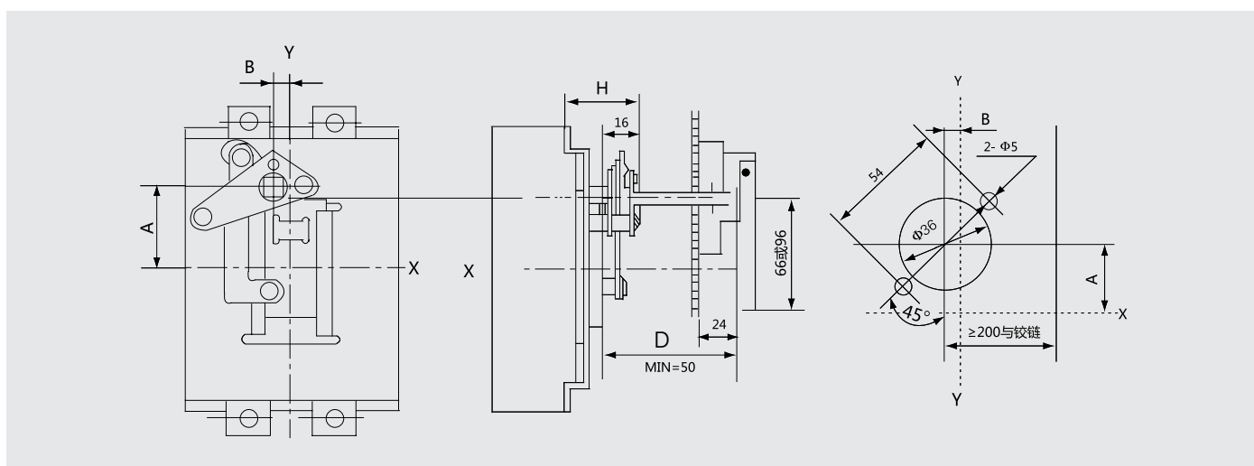
CS2-A型手柄安装开孔示意图
