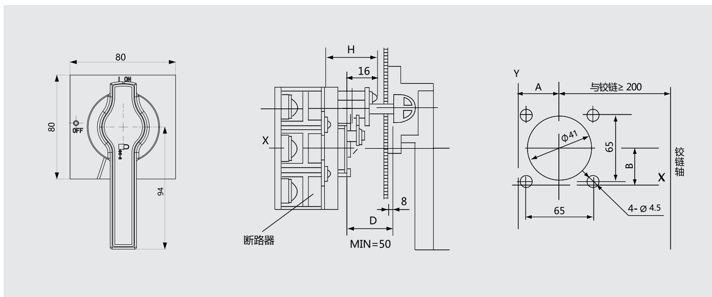
IP65手柄（400壳架以上）开孔示意图
