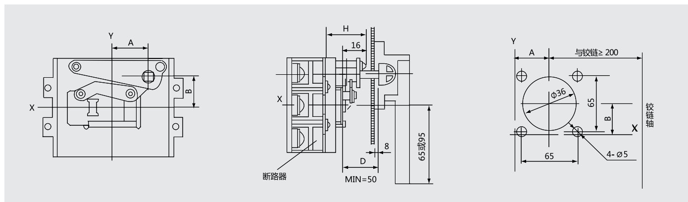
IP65手柄（250壳架以下）开孔示意图
