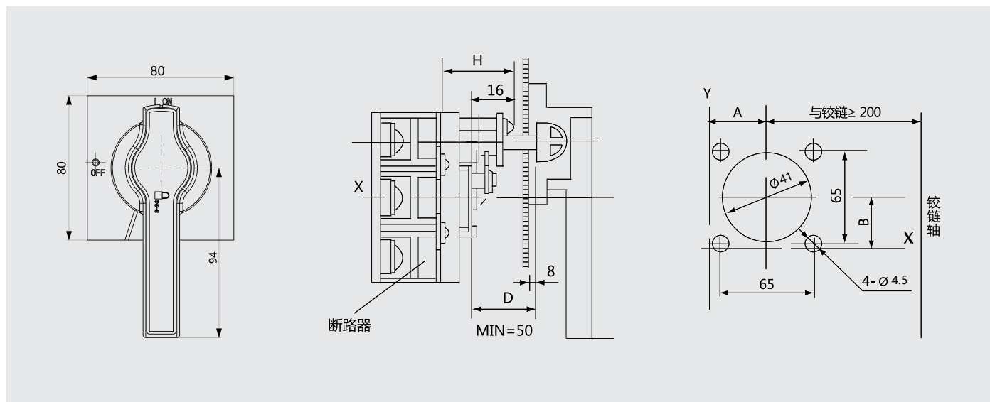
P65手柄（400壳架以上）开孔示意图
