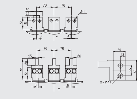
详图
