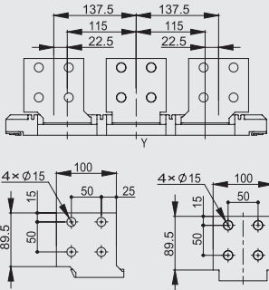
详图
