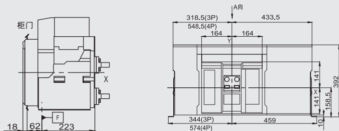
尺寸
