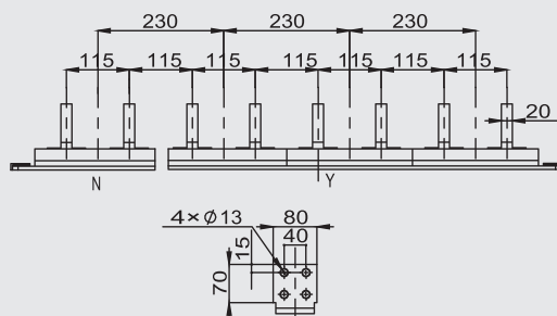
详图
