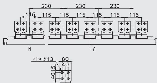
详图
