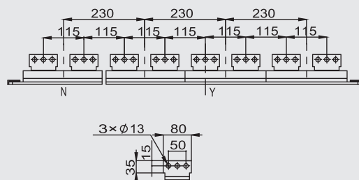
详图
