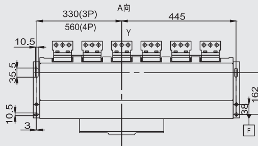
固定详图
