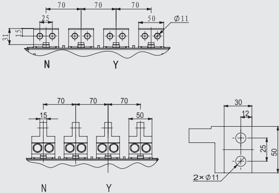
详图
