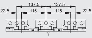
详图
