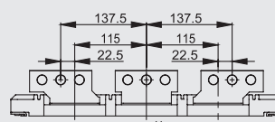
详图
