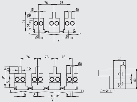
详图
