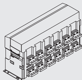
水平接线
