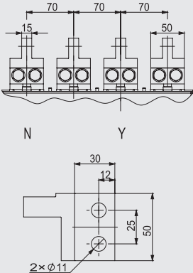
固定详图
