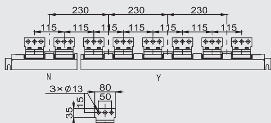
详图
