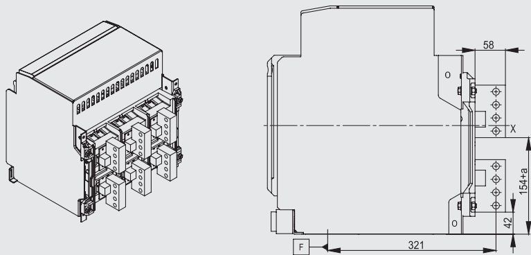
垂直接线
