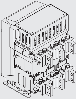
垂直接线
