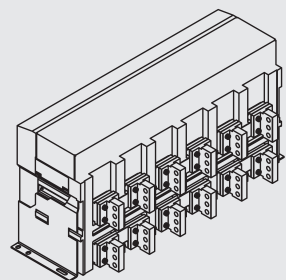
垂直接线
