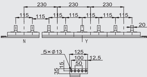
详图
