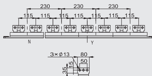
详图
