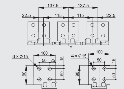
详图
