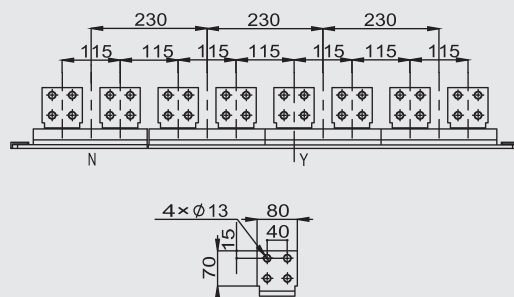
详图
