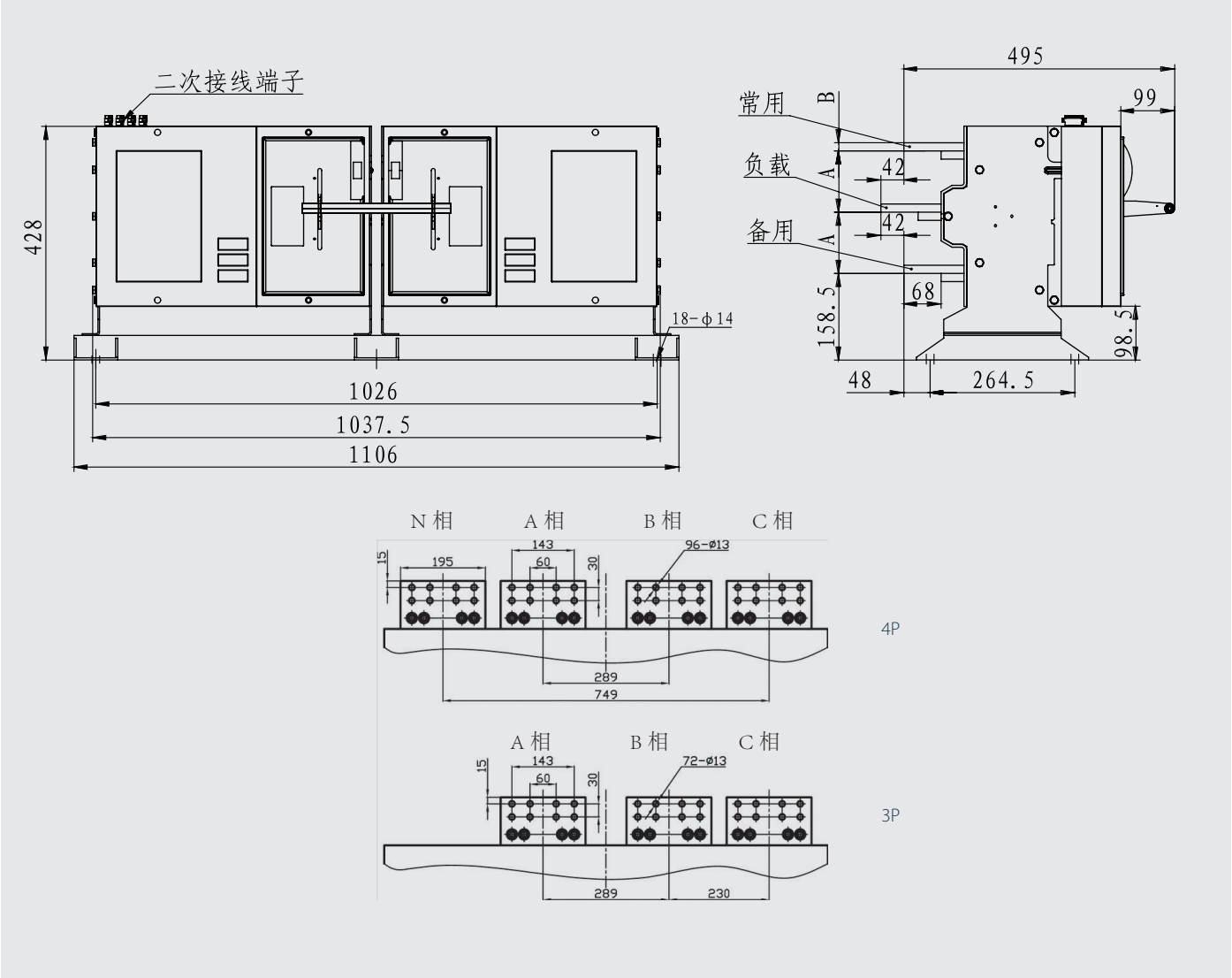
◆ NDQ3H-5000机构本体外形尺寸和安装尺寸
