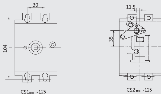
配NDM3E-125的手操机构
