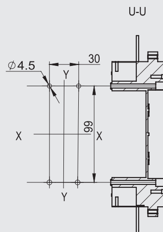
插入式板前接线安装板开孔尺寸
