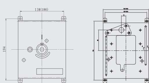
配NDM3E-400的手操机构
