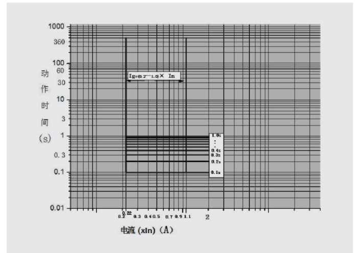
NDM3EX-1600 接地保护特性曲线
