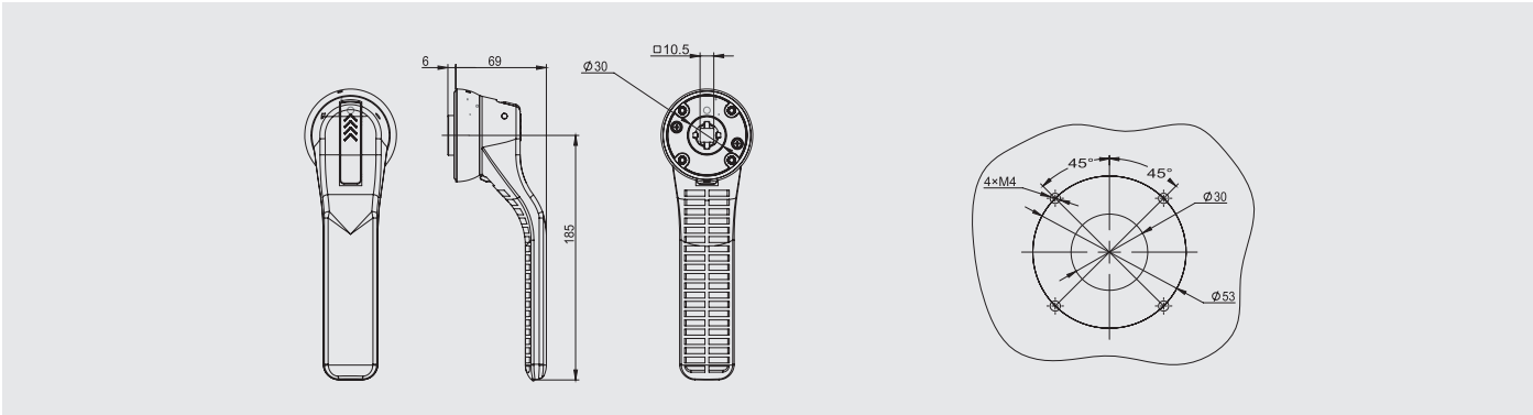
NDM3EX-1600 尺寸
