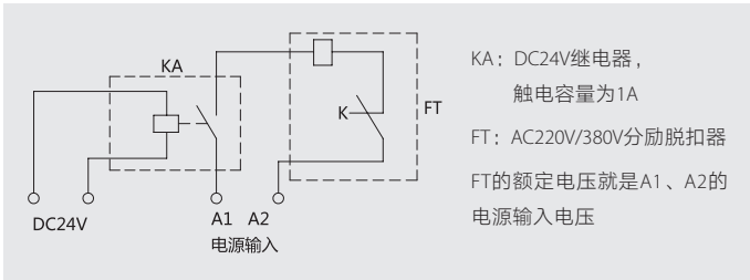
分励脱扣器电气特性
