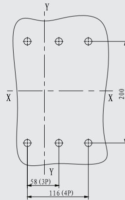
三极/四极
