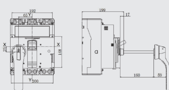
配NDM3EX-1600的手操机构
