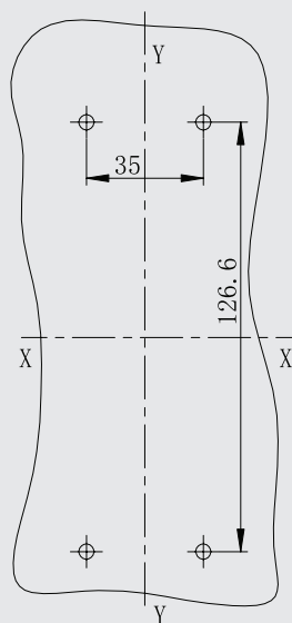
板前接线安装板开孔尺寸
