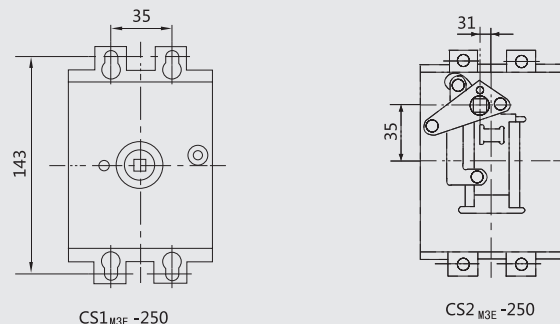
配NDM3E-250的手操机构
