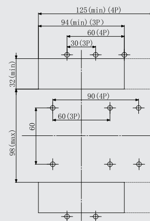
插入式板后接线安装板开孔尺寸
