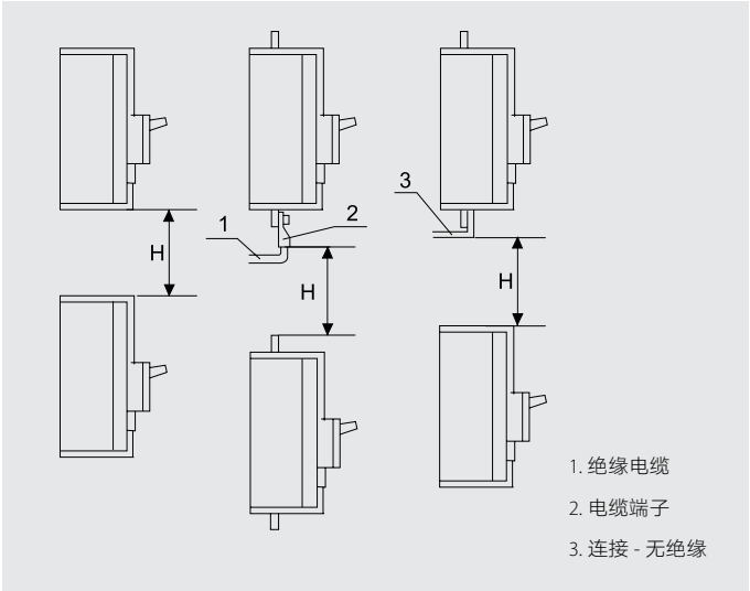
断路器叠装之间最小距离
