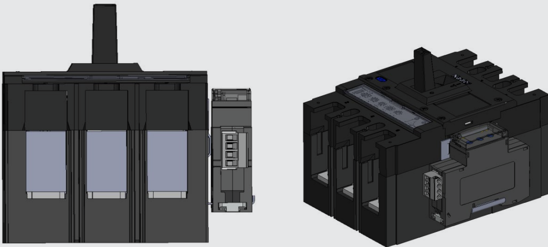
通讯型断路器与通讯适配器连接图
