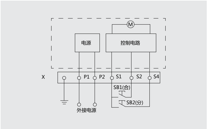
接线图（虚框内为断路器外部附件接线图）
