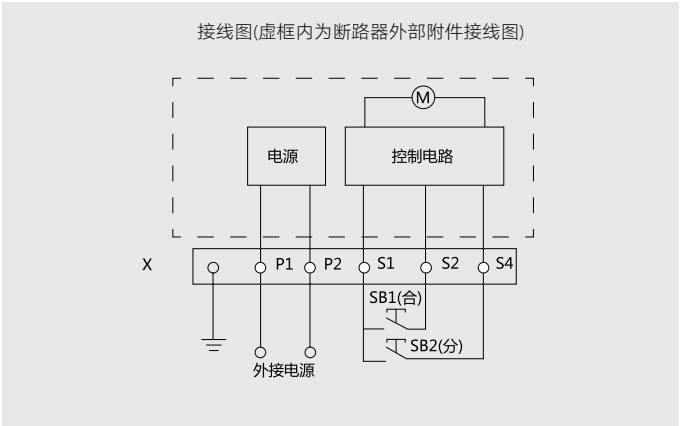
电动操作机构（配用NDM2Z-63~630系列）
