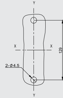
板前接线安装板开孔尺寸
