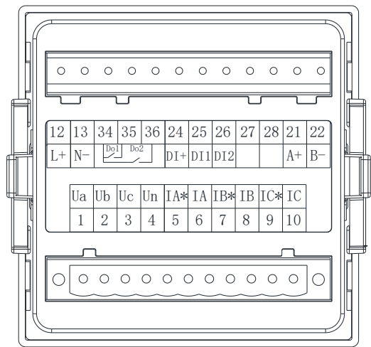
图 4 接线端子图
