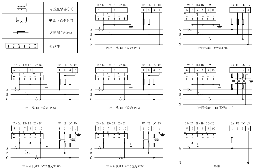
图 5 典型接线图
