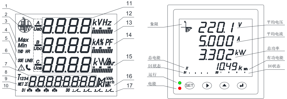
图 6 液晶屏示意图
