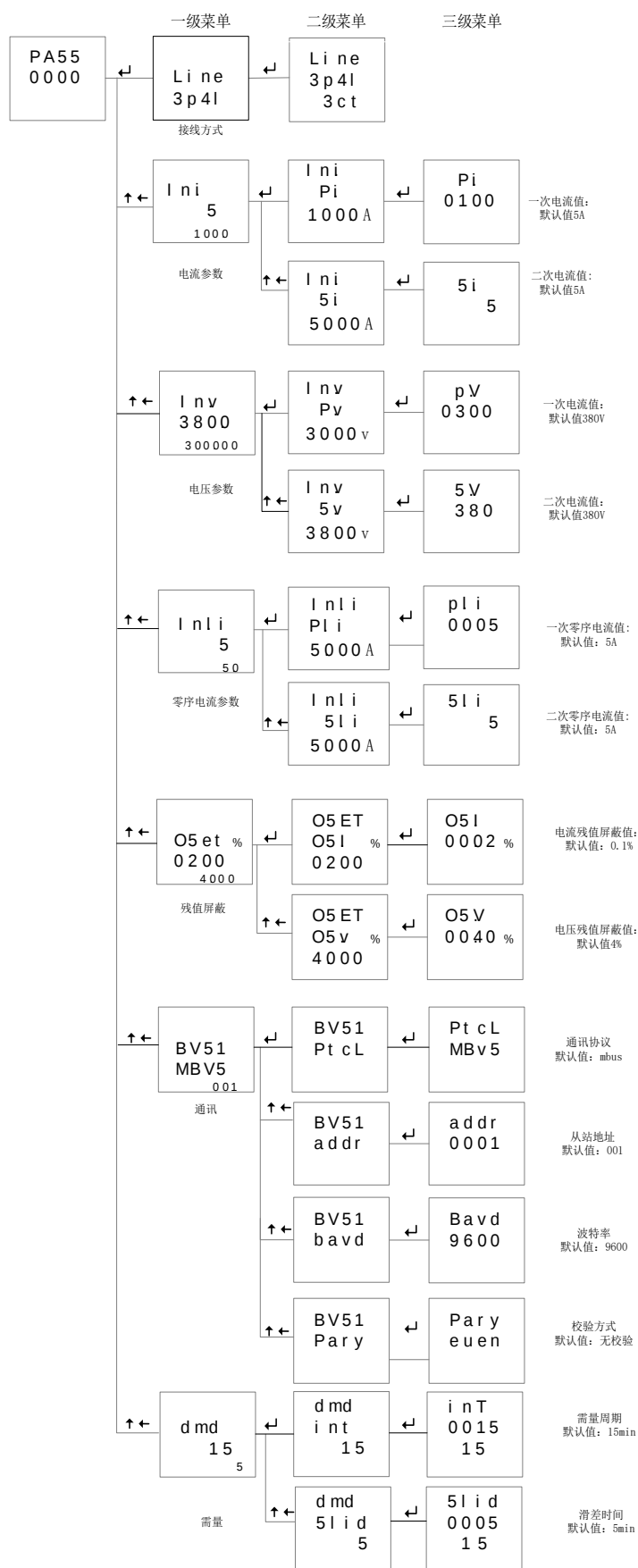
图 17 电流、电压、通讯及需量参数设置
