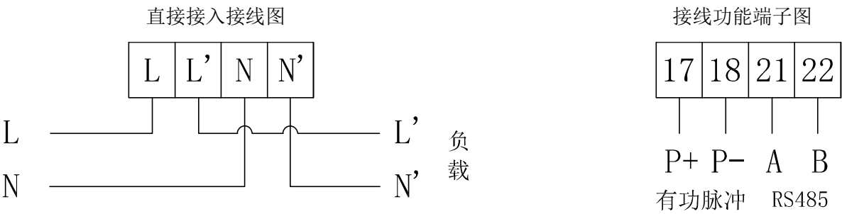
图 8 接线端子图
