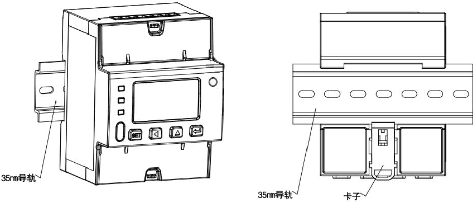
图 4 产品导轨安装示意图
