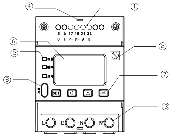
图 6 设备俯视图
