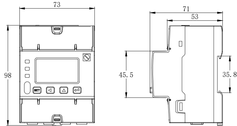
图 2 RS485 通讯产品外形尺寸
