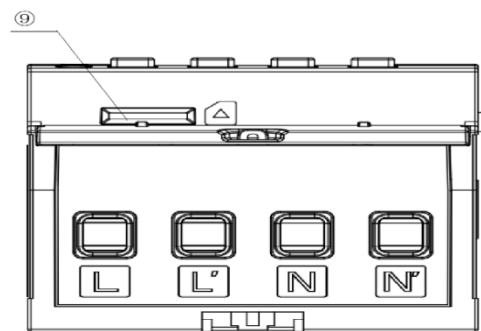
图 7 设备侧视图
