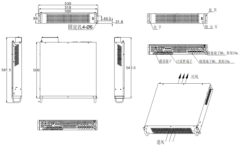
图 2-1 SVG-50K 模块外形尺寸图
