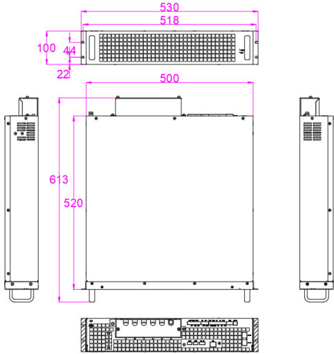
图 2-1 (1) 150A APF 机架式 LED 功率模块安装尺寸图
