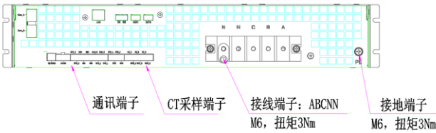
图 2-4 (2) 150 APF 模块接线端子示意图
