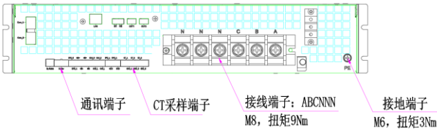
图 2-4 (1) 150 APF 模块接线端子示意图
