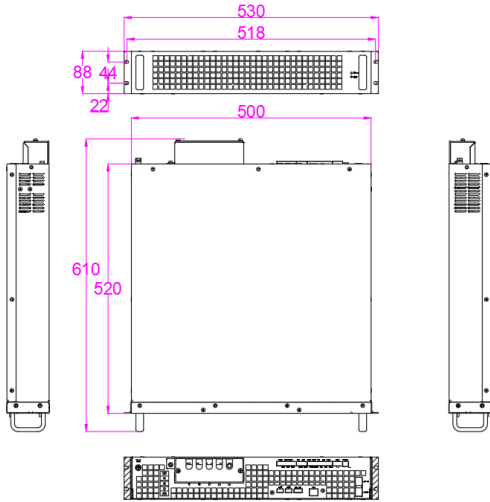
图 2-1 (2) 100A APF 机架式 LED 功率模块安装尺寸图
