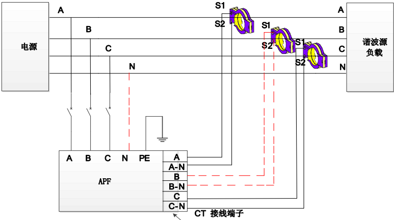
图 2-3 100/150 APF 单功率模块配线及安装框图
