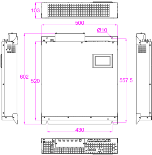
图 2-2 (1) 150A APF 壁挂式功率模块安装尺寸图
