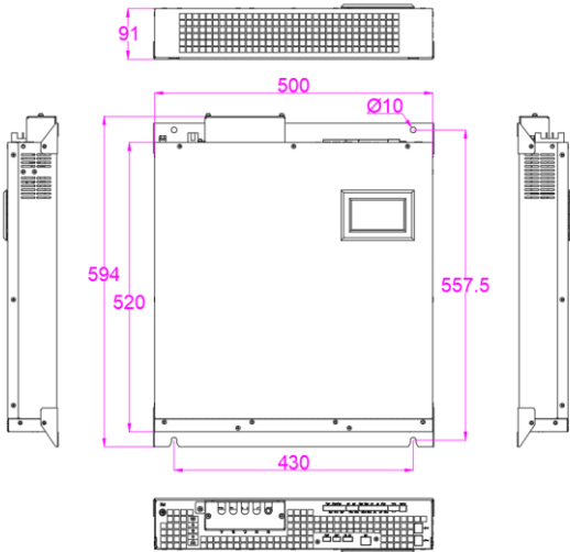
图 2-2 (2) 100A APF 壁挂式功率模块安装尺寸图
