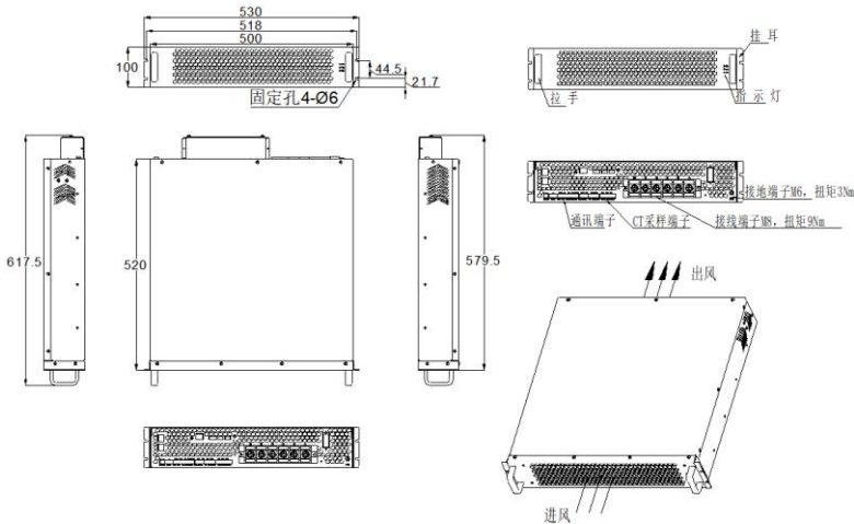
图 2-1 APF-150A 模块外形尺寸图
