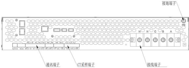
图 2-3 端口配线图
