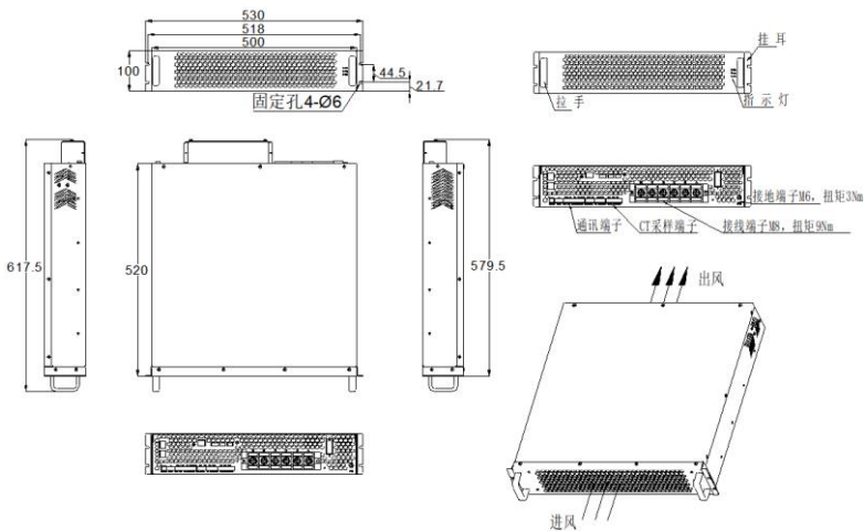
图 2-1 SVG-100K 模块外形尺寸图
