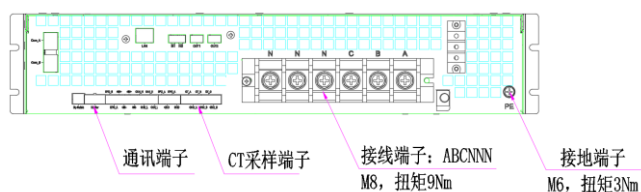
图 2-4 (1) 100 SVG 模块接线端子示意图
