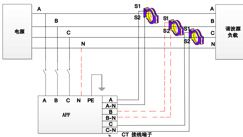
图 2-3 100 SVG 单功率模块配线及安装框图
