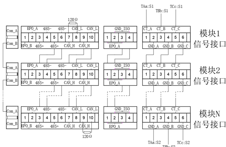
图 2-7 多模块并机网侧 CT 信号接口接线图
