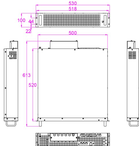
图 2-1 SVG 机架式 LED 功率模块安装尺寸图
