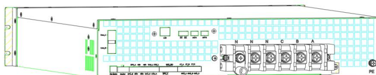
图 2-4 100 SVG 模块背部示意图
