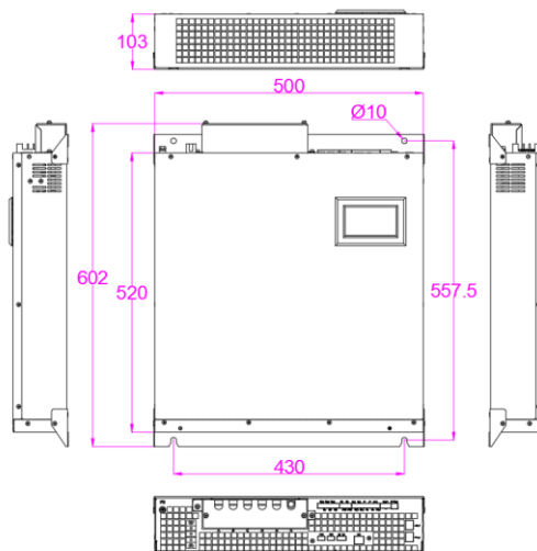
图 2-2 SVG 壁挂式 LCD 功率模块安装尺寸图
