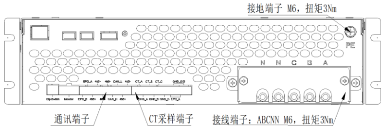
图 2-3 端口配线图
