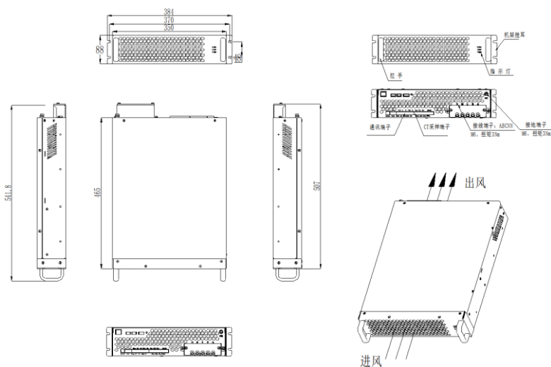
图 2-1 APF-50A 模块外形尺寸图
