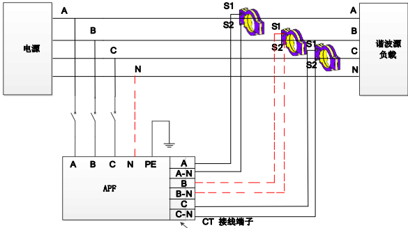
图 2-2 单功率模块配线及安装框图
