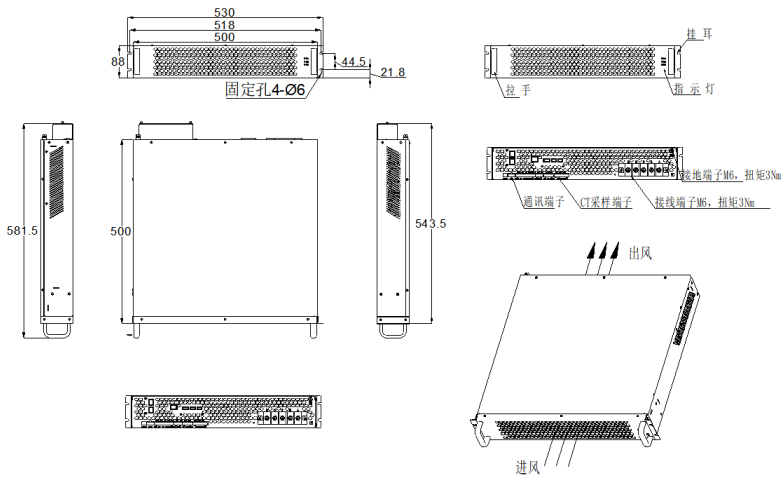
图 2-1 APF-100A 模块外形尺寸图
