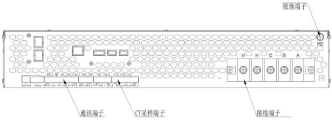
图 2-3 端口配线图
