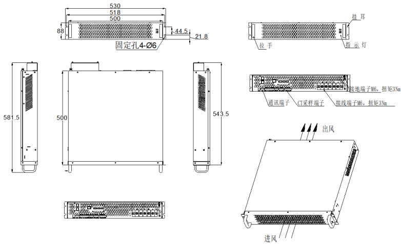
图 2-1 APF-75A 模块外形尺寸图
