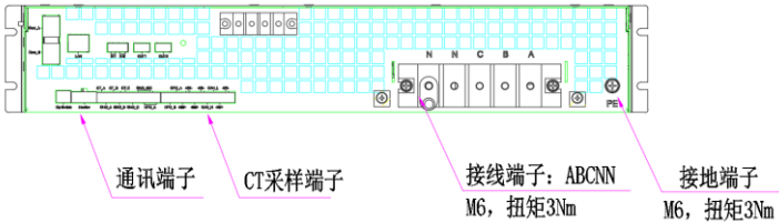
图 2-4 (1) 50 SVG 模块接线端子示意图
