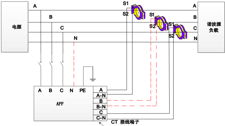
图 2-3 50 SVG 单功率模块配线及安装框图
