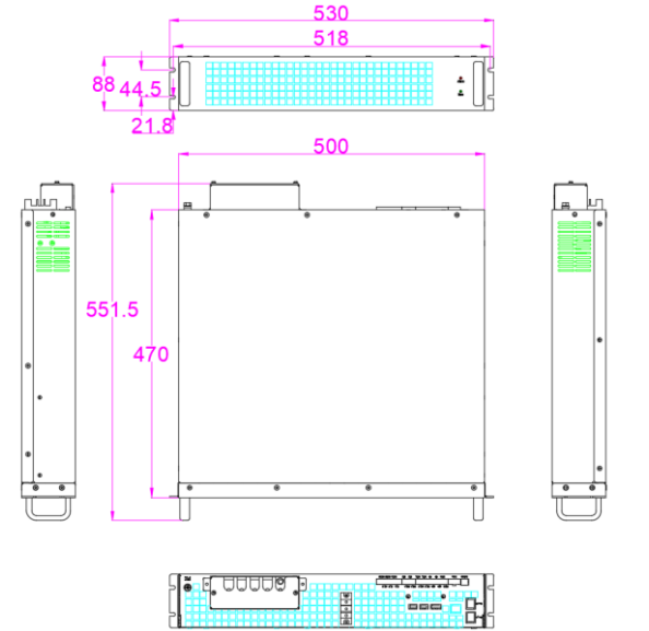
图 2-1 SVG 机架式 LED 功率模块安装尺寸图
