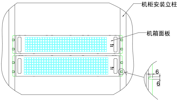
图 2-3 机架模块安装示意图
