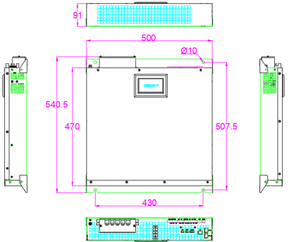
图 2-2 SVG 壁挂式 LCD 功率模块安装尺寸图
