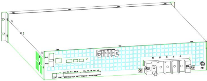
图 2-4 50 SVG 模块背部示意图
