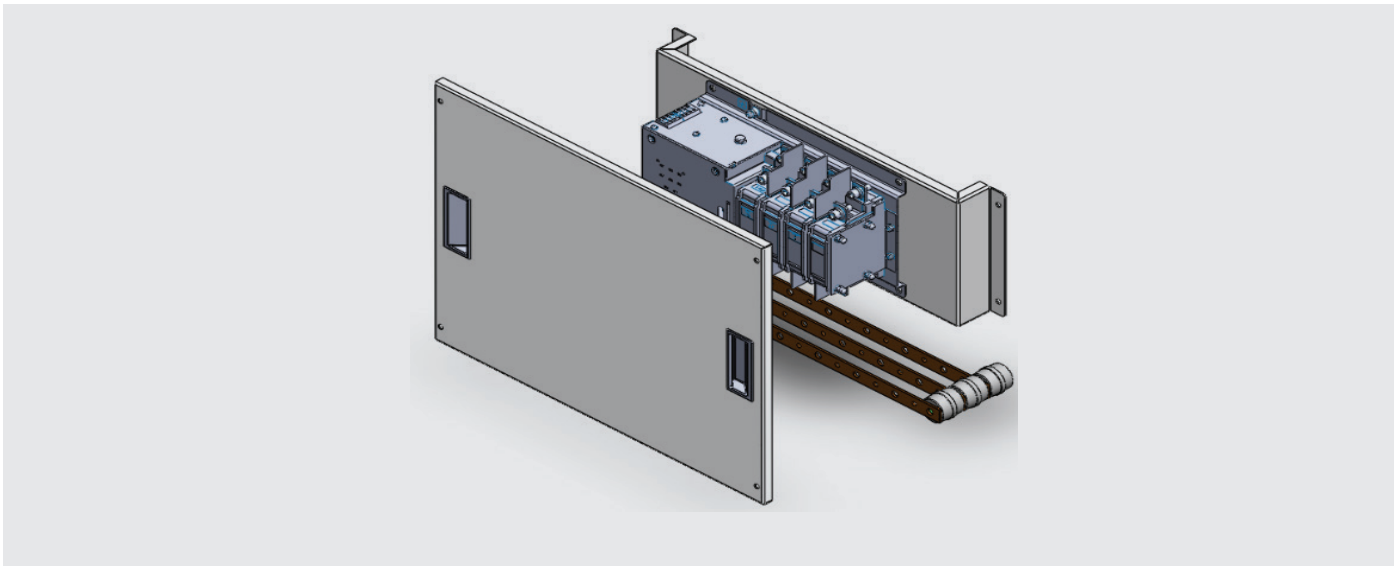
NDQ3H 双电源模块
