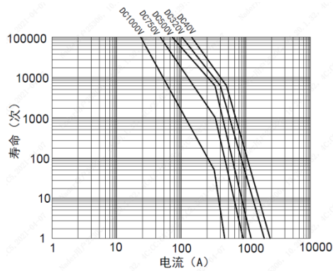
NDZ3W-250
