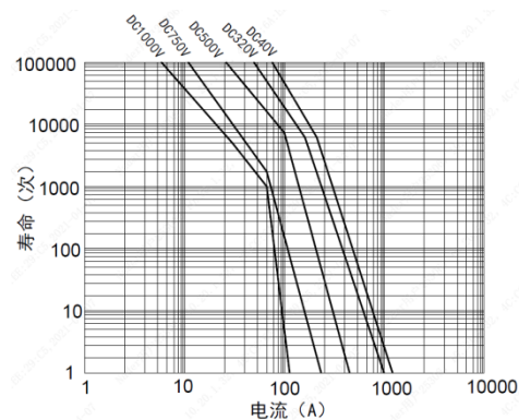
NDZ3W-100
