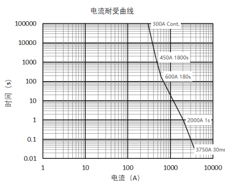
NDZ3W-300
