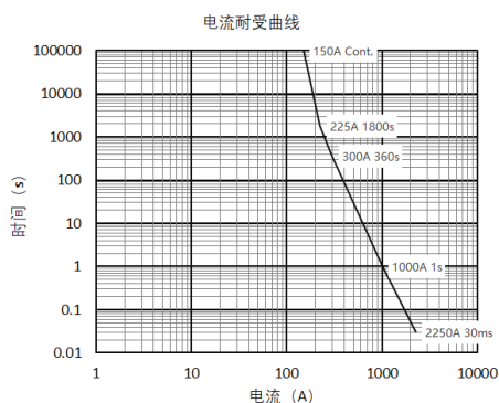
NDZ3W-150
