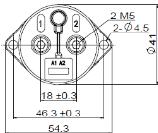
NDZ3W-50/100
