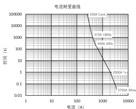
NDZ3W-250
