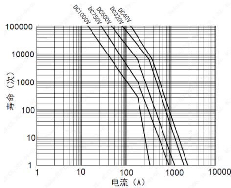
NDZ3W-150
