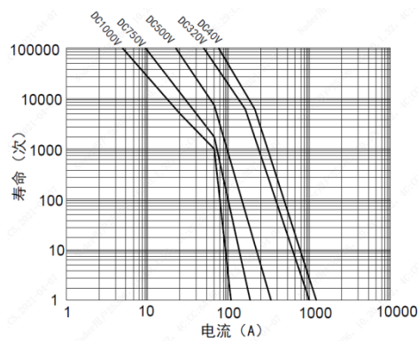
NDZ3W-50
