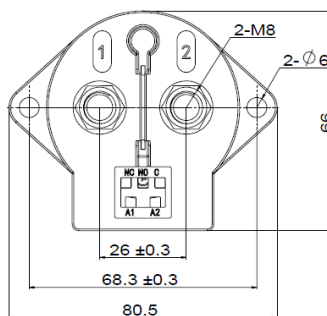
NDZ3W-150/200/250/300
