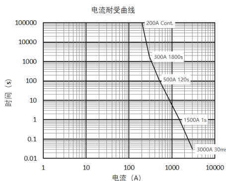
NDZ3W-200
