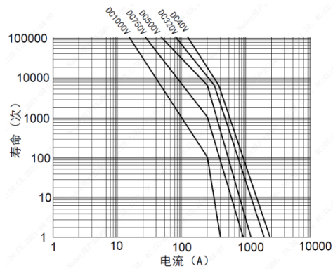
NDZ3W-200
