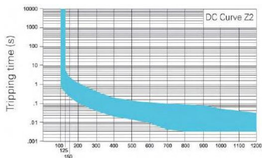
Z2 Curve
