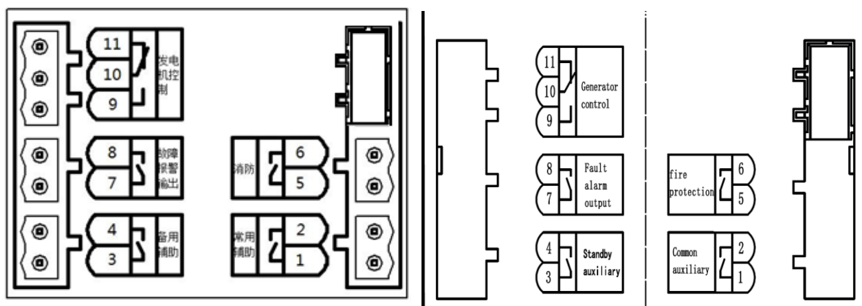
基本型外部端子接线图
