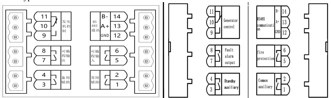
D 型外部端子接线图
