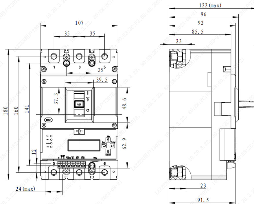
250-3P External Dimensions
