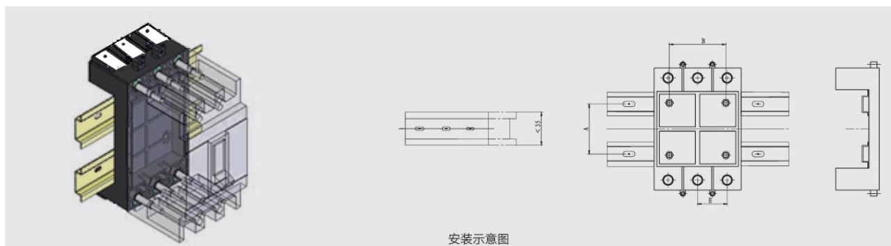
安装示意图
